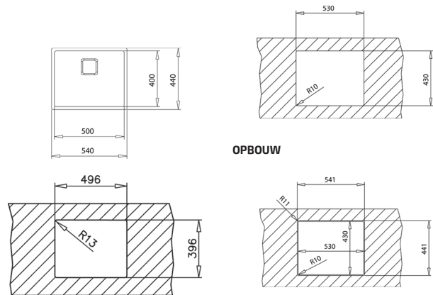
VLAKKE INBOUW
