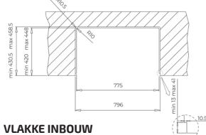
VLAKKE INBOUW
