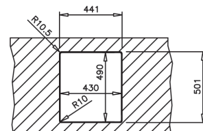
VLAKKE INBOUW
