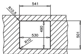
VLAKKE INBOUW
