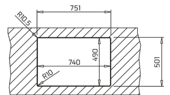
VLAKKE INBOUW
