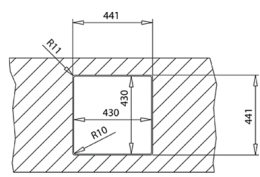
VLAKE INBOUW
