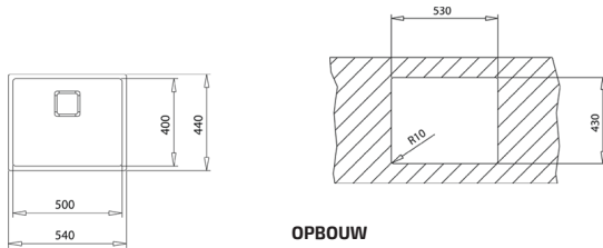
OPBOUW
