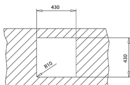
OPBOUW
