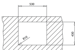
OPBOUW
