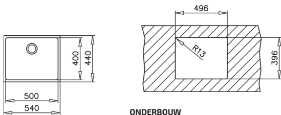
ONDERBOUW
