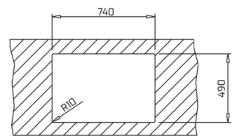
OPBOUW
