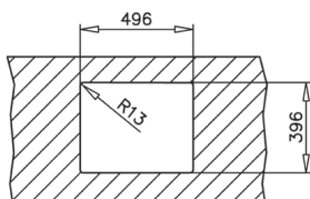
ONDERBOUW
