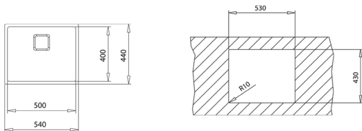
OPBOUW
