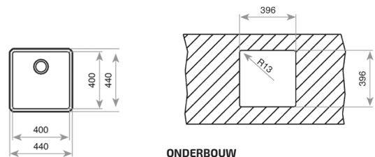
ONDERBOUW
