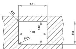
VLAKKE INBOUW
