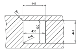
VLAKKE INBOUW
