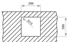
ONDERBOUW
