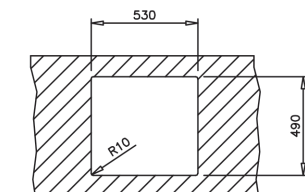
OPBOUW
