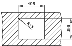
ONDERBOUW
