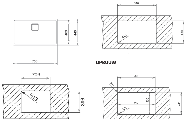
VLAKKE INBOUW
