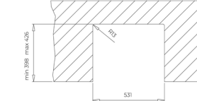
ONDERBOUW
