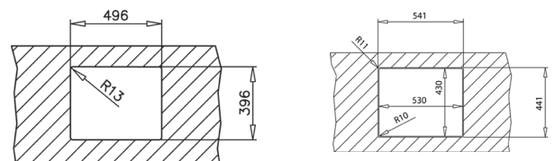
ONDERBOUW
