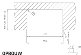
OPBOUW
