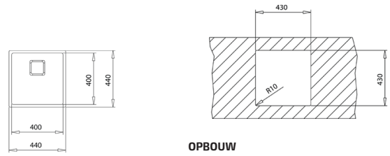
OPBOUW
