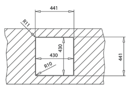
VLAKKE INBOUW
