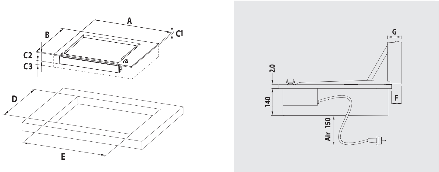
DISEGNO TECNICO 3
