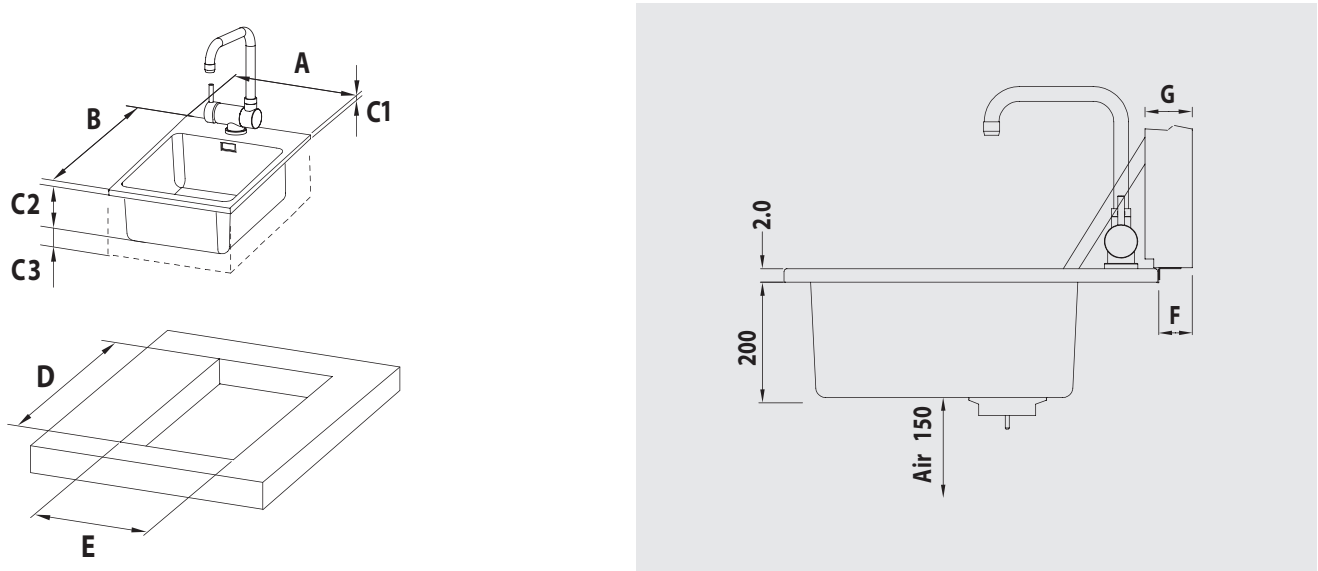
DISEGNO TECNICO 6
