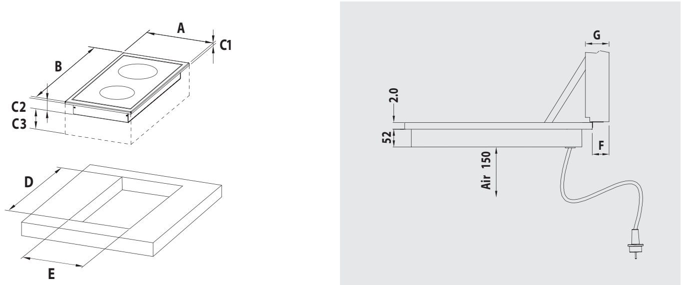
DISEGNO TECNICO 5
